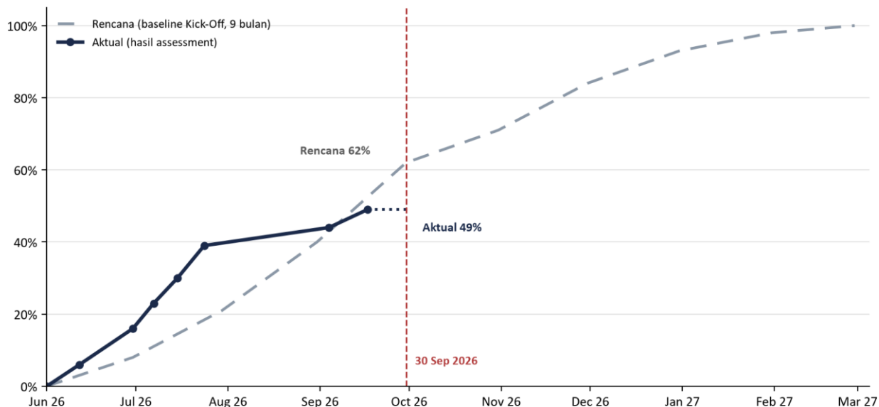
Gambar 1. Kurva-S proyek — rencana vs aktual, per 30 September 2026.
